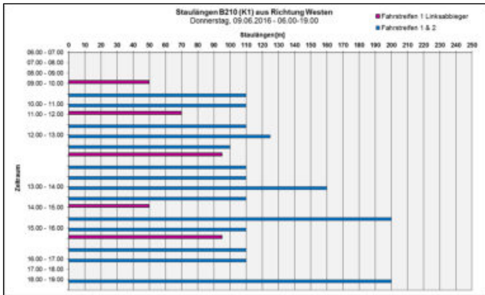
Abb. 3.9 K 1 Emder Straße / Auricher Straße / Norder Straße Staulängen Emder Straße aus Richtung Westen
