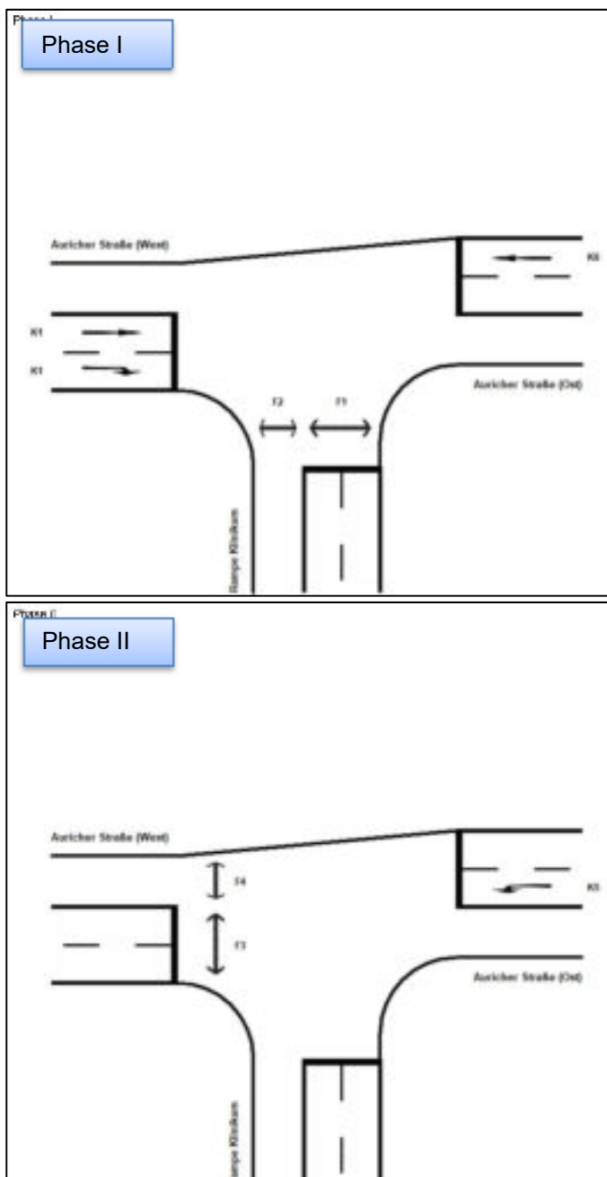
Abb. 6.8 Phasenablauf (Phasen I und II)
