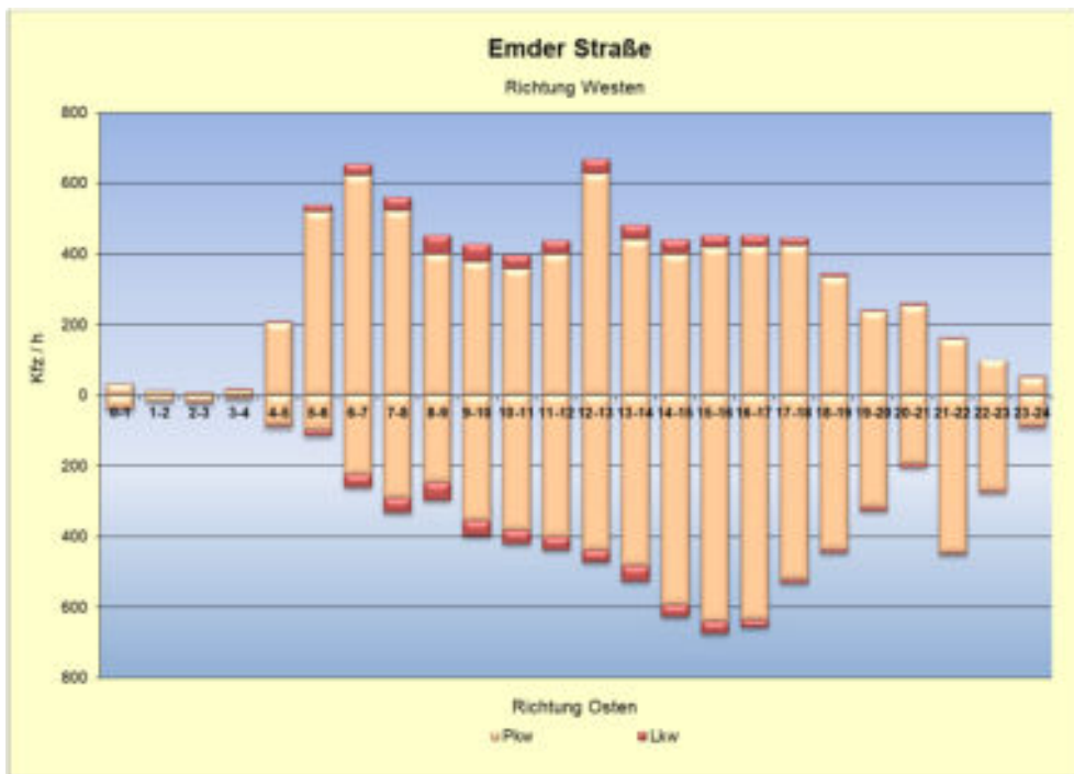
Abb. 3.5 Tagesganglinie Emders Straße (B 210) westlich B 72 (Donnerstag, 09.06.2016)
