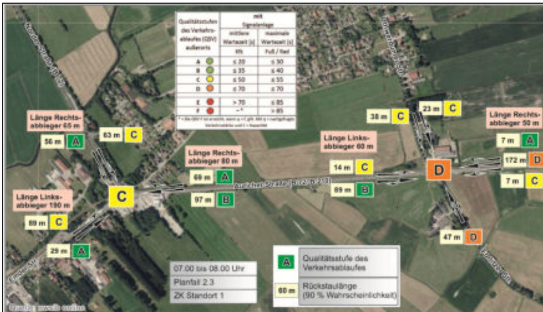
Abb. 5.11 Standorte 1 und 2: Qualität der Verkehrsanlagen gemäß HBS 2015 (Planfall P 2.3 plus ZKG)
