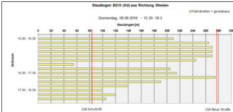
Abb. 3.11 K 4 Auricher Straße / Ekelser Straße Staulängen Auricher Straße aus Richtung Westen
