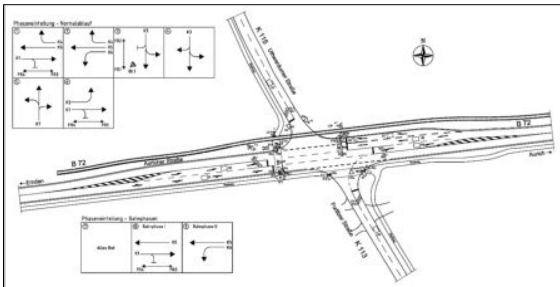
Abb. 5.13 Lageplan Knotenpunkt B 72/B210 / K 113 / K 115
