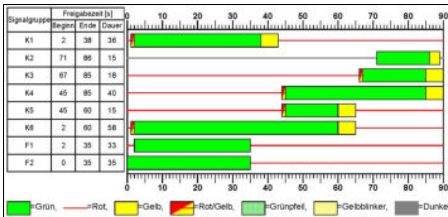
Abb. 6.12 Signalzeitenplan 07 bis 08 Uhr ohne Fußgängerquerung der B 72 / B 210
