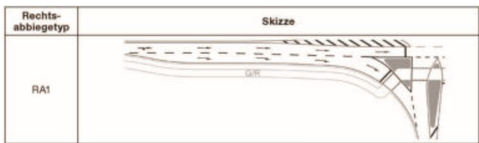
Abb. 6.2 Systemskizze Rechtsabbiegetyp RA 1
