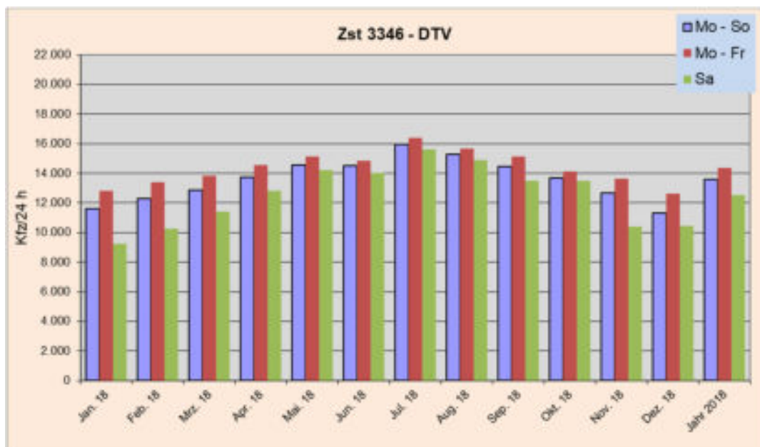
Abb. 3.2 Verkehrsmengen B 72 (Zst. 3346) im Jahr 2018
