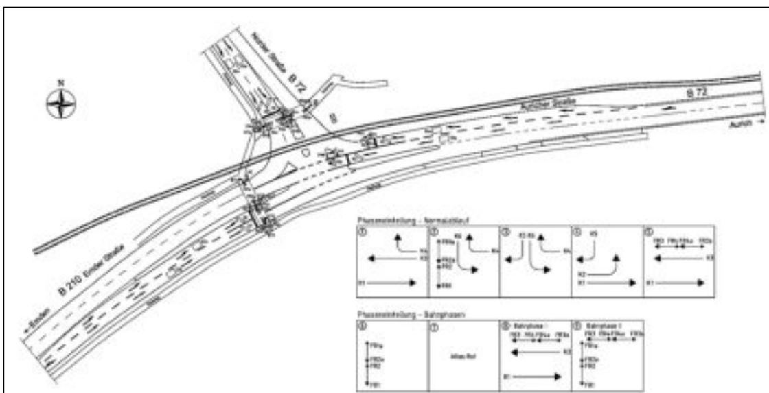
Abb. 5.10 Lageplan Knotenpunkt B 72 / B 210 in Georgsheil
