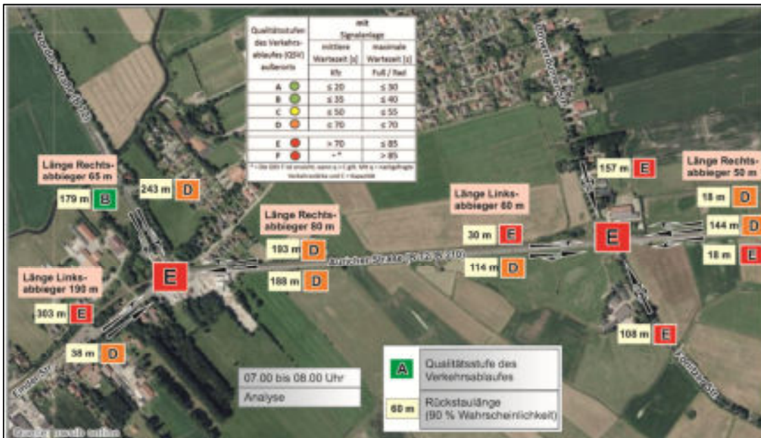
Abb. 5.9 Analyse Qualität der Verkehrsanlagen Simulation mit Zugverkehr - 07:00 bis 08:00 Uhr
