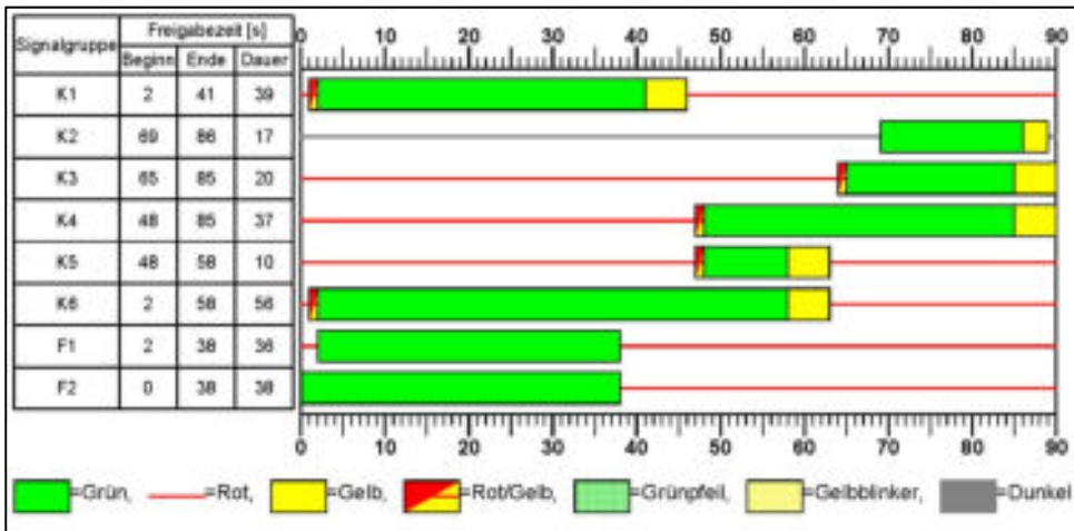
Abb. 6.15 Signalzeitenplan 16 bis 17 Uhr ohne Fußgängerquerung der B 72 / B 210
