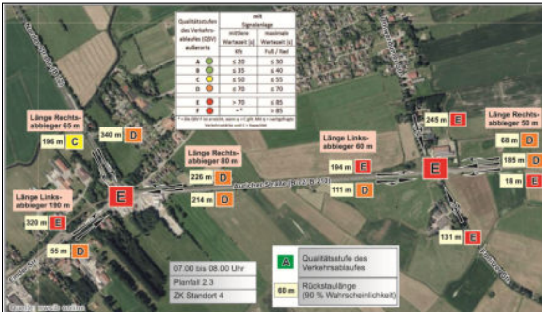
Abb. 5.15 Standorte 3 und 4: Qualität der Verkehrsanlagen Simulation mit Zugverkehr (Planfall P 2.3 plus ZKG)
