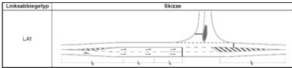
Abb. 6.1 Systemskizze Linksabbiegetyp LA 1
