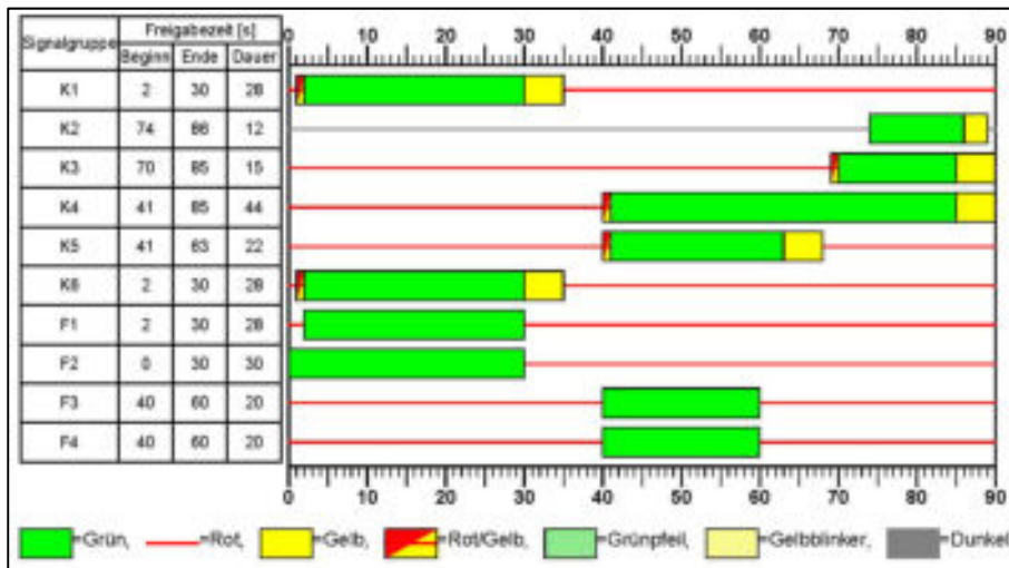
Abb. 6.11 Signalzeitenplan 07 bis 08 Uhr mit Fußgängerquerung der B 72 / B 210
