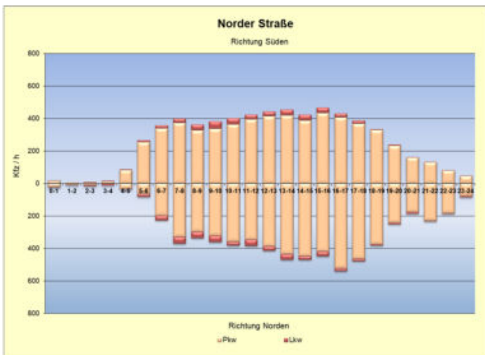
Abb. 3.6 Tagesganglinie Norder Straße (B 72) (Donnerstag, 09.06.2016)
