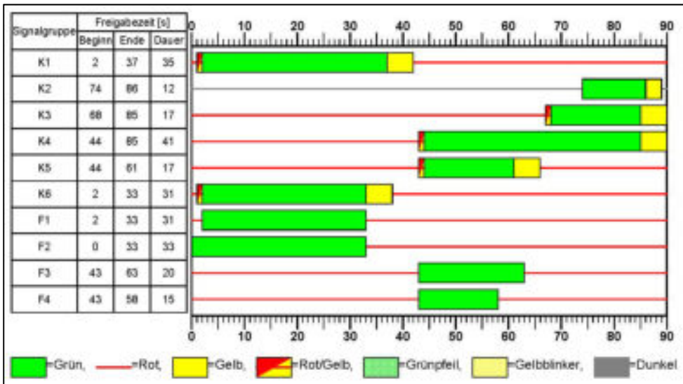
Abb. 6.14 Signalzeitenplan 16 bis 17 Uhr mit Fußgängerquerung der B 72 / B 210
