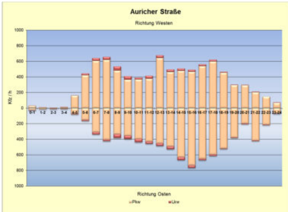
Abb. 3.7 Tagesganglinie Auricher Straße (B 210) östlich B 72 (Donnerstag, 09.06.2016)
